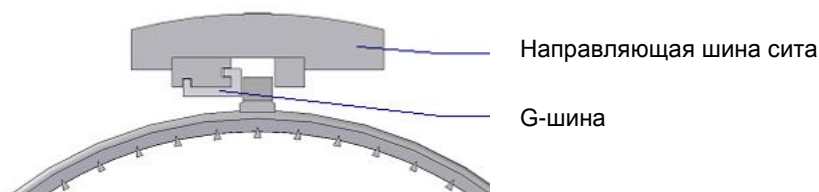
Рис. 13-4 G-шина
