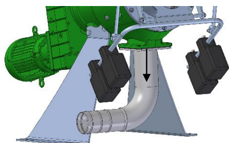
Рис.4-8 Сливное колено
