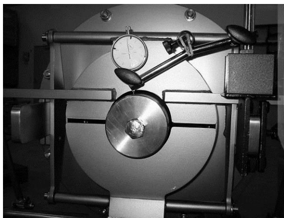
Рис. 13-12: Контроль осевого биения шнека
