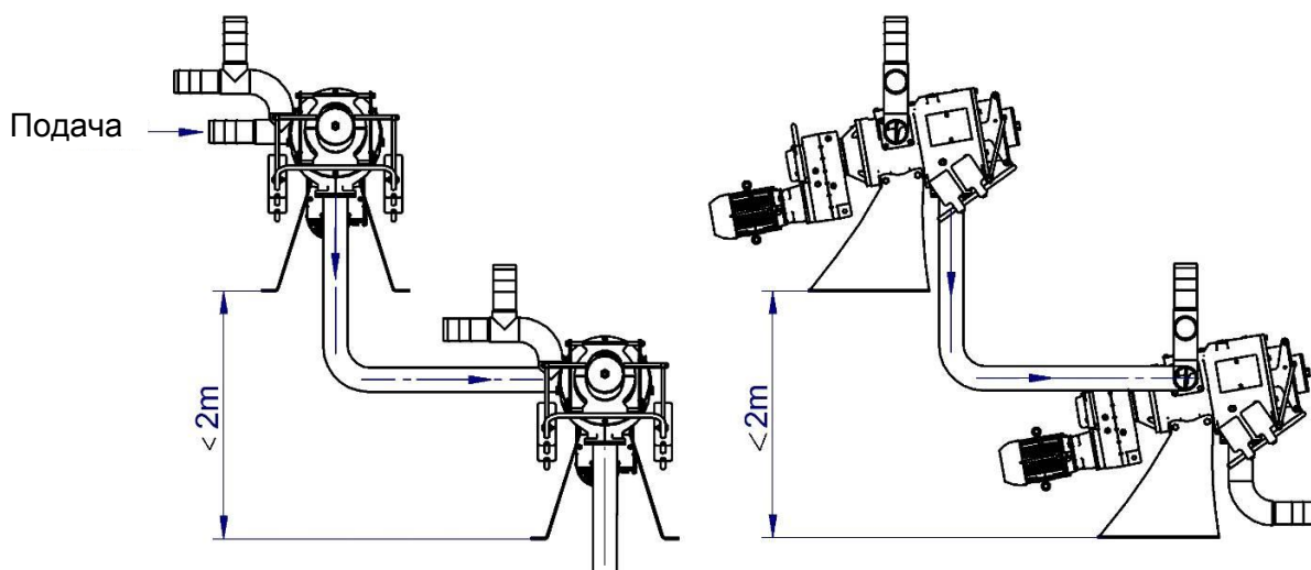
Рис. 10-1 Типичное расположение при последовательном подключении 2 сепараторов
