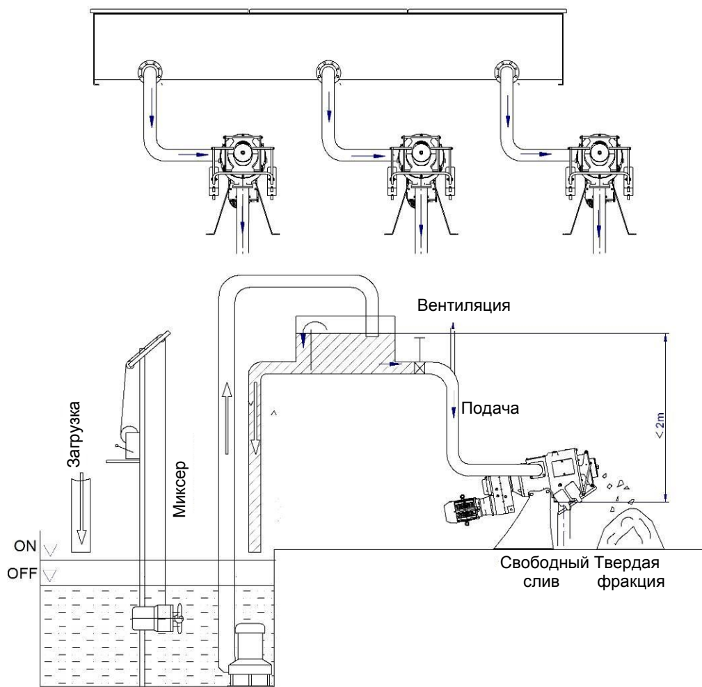
Рис. 9-1. Типичное расположение при параллельном включении 3 сепараторов
