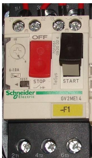
Рис. 15-3 Защита двигателя F1
