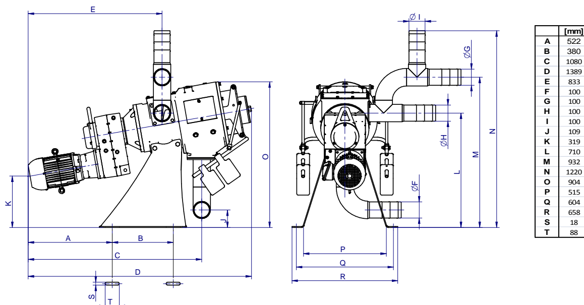
Рис. 4-3 Размеры сепаратора Compact
