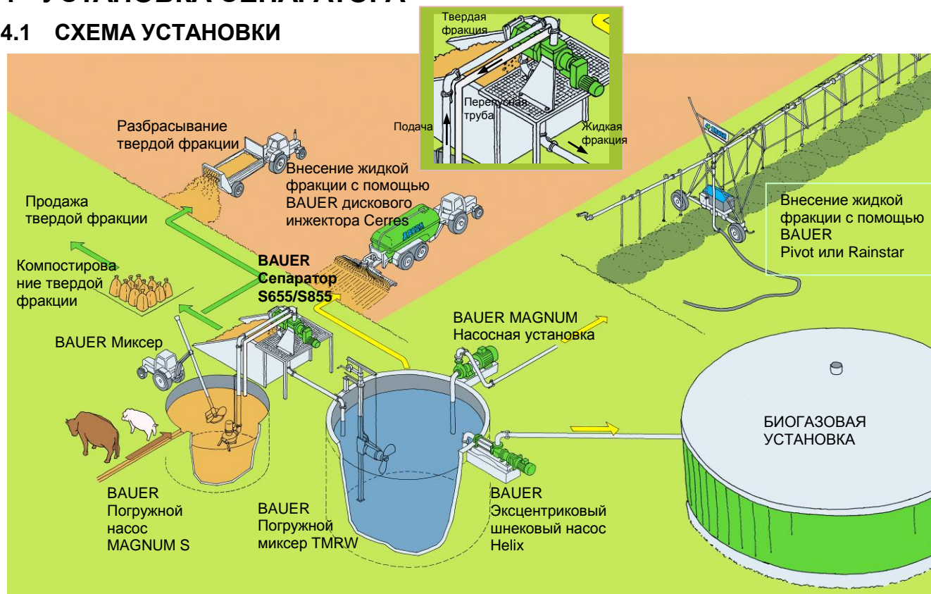
Рис. 4-1 Схема установки
