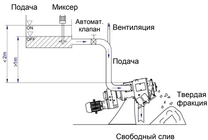
Рис.4-6 Загрузка самотеком из вышележащей накопительной емкости
