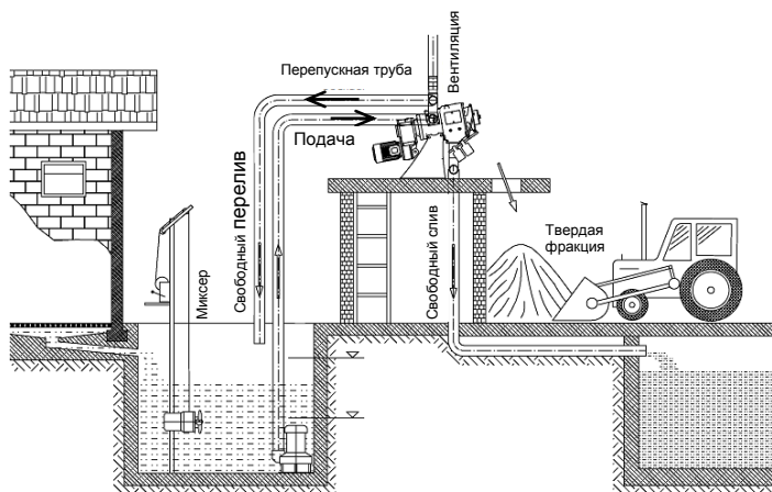
Рис.4-5 Загрузка насосом
