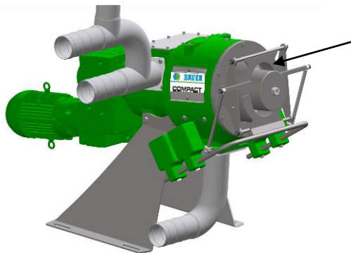
Рис. 7-2 Выходные створки
