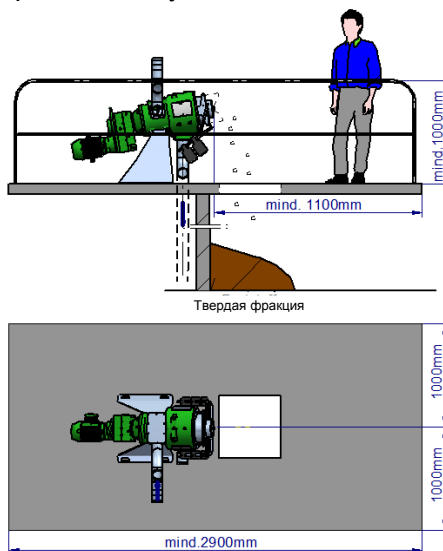
Рис. 4-4 Определение размеров монтажной площадки
